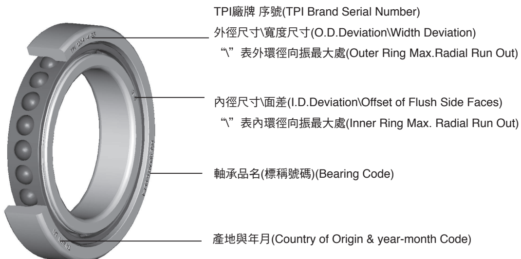
圖2-1 軸承的記號與說明
