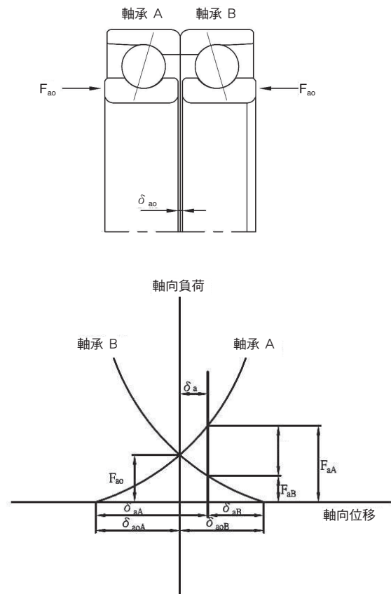
圖5-2 預壓負荷示意圖
